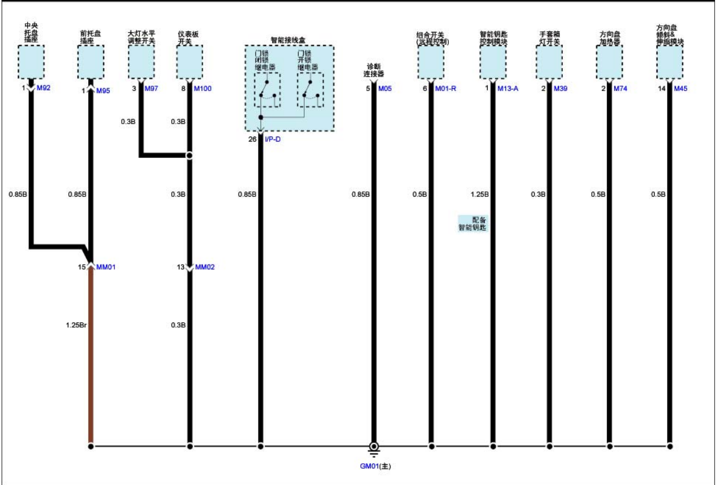
搭铁分布 (1)
